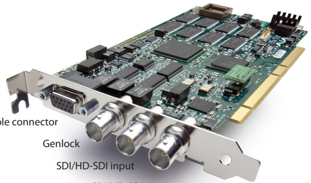
SDI/HD-SDI output
